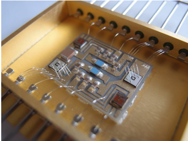
Module utilisé pour réaliser des convertisseurs pouvant fonctionner à des hautes températures. ©Laboratoire AMPERE
