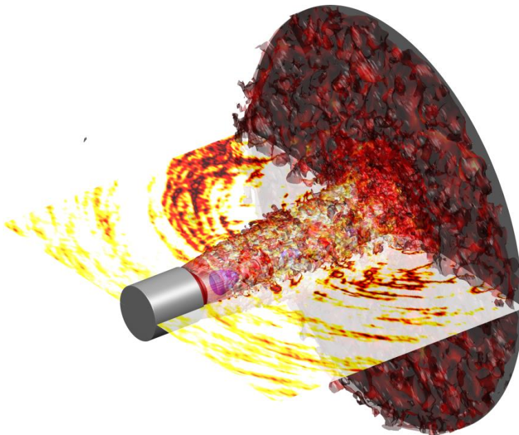
Simulation numérique directe du bruit émis par un jet supersonique impactant un obstacle. ©Daniel Juvé
